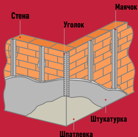
Профиль угловой
